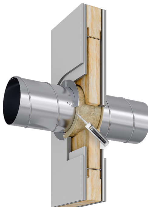
FLE60 flange
