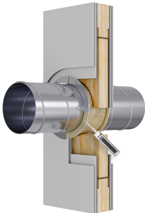
FL flange
