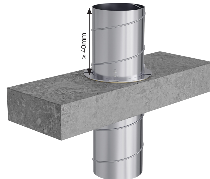
FLE60 flange
